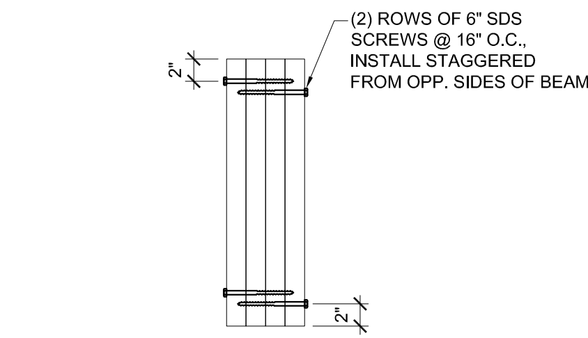
17 DETAIL SCALE: NO SCALE
