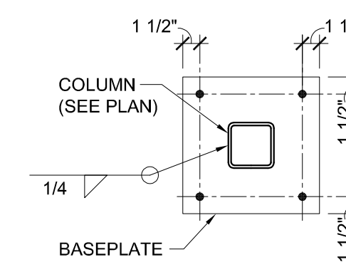
14 BASEPLATE DETAIL SCALE: NO SCALE
